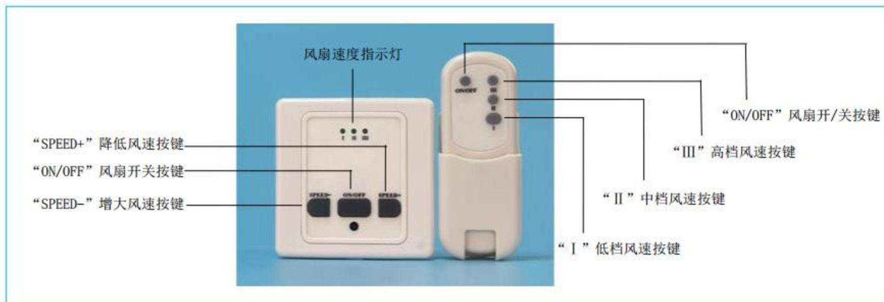
开关面板区域各按键功能示意图
