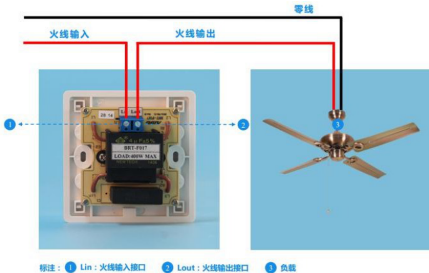
图四 单火线接线示意图
