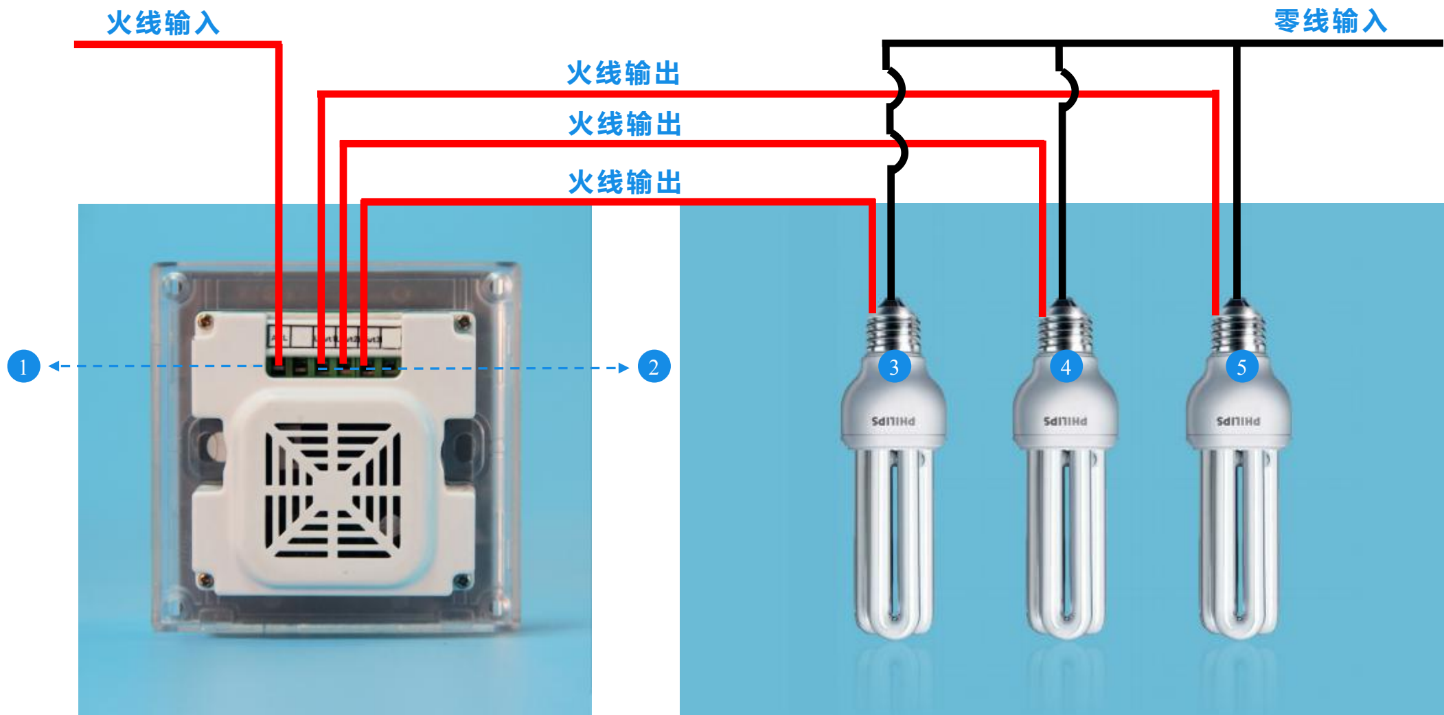
标注：① ACL：火线输入接口 ② Lout：火线输出接口 ③ ④ ⑤ 负载（灯具）
