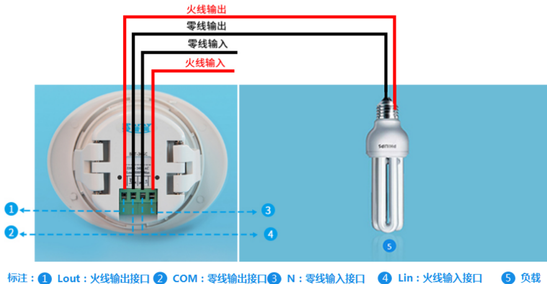
图六 BRT-306C 接线图
